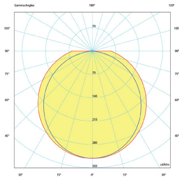
Winkelverteilung der Leuchtdichte.
